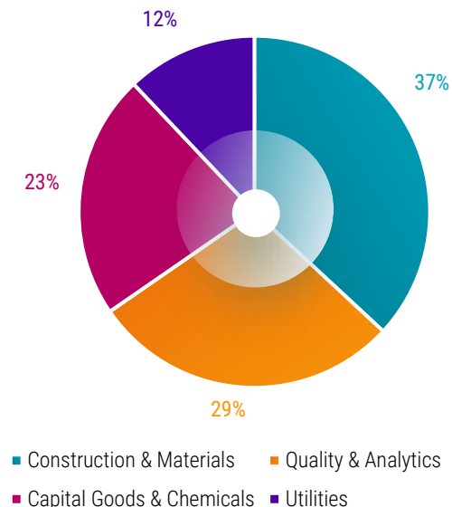
Clusterverteilung
