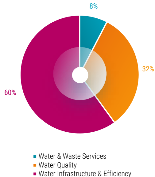
Clusterverteilung
