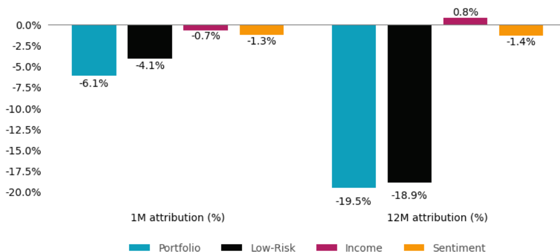
Figuur 1 – Factorattributie
