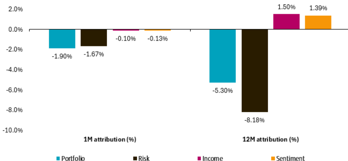
Figuur 1 – Factorattributie
