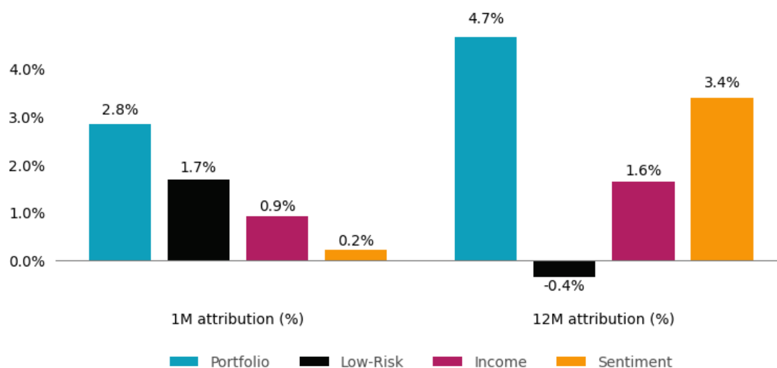
Figuur 1 – Factorattributie
