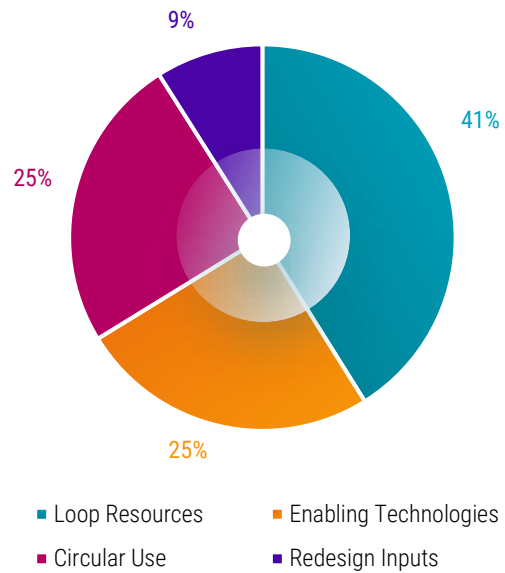
Clusterverteilung
